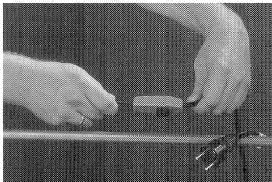
De verwarmingskabel wordt gestrekt langs de leiding aangelegd.
